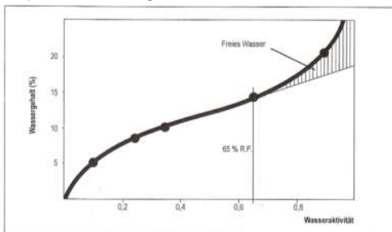
Abb. 11-II: Sorptionsisotherme von Getreide (W. Klingler)
